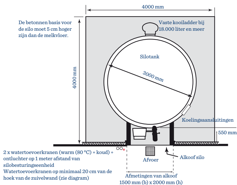
Afmetingen van de Mueller® Silo bovenaanzicht
