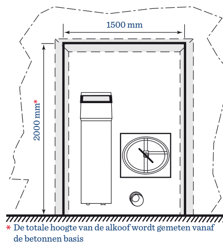
Afmetingen van de Mueller® Silo Alcove vooraanzicht
